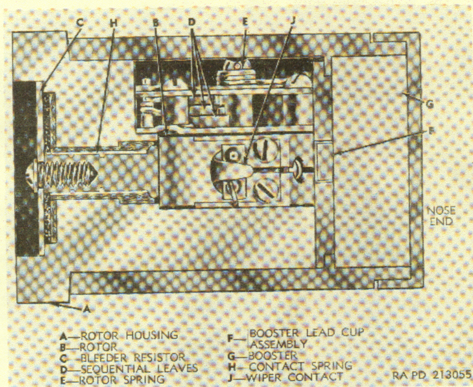
Figure 25. Fuze, PIBD: M509.
