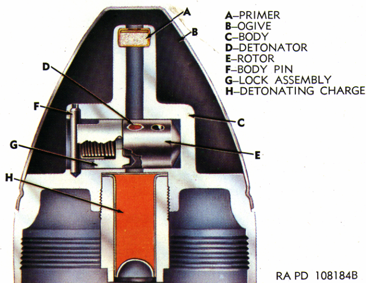
Figure 24. Fuze, PI: M90A1.
